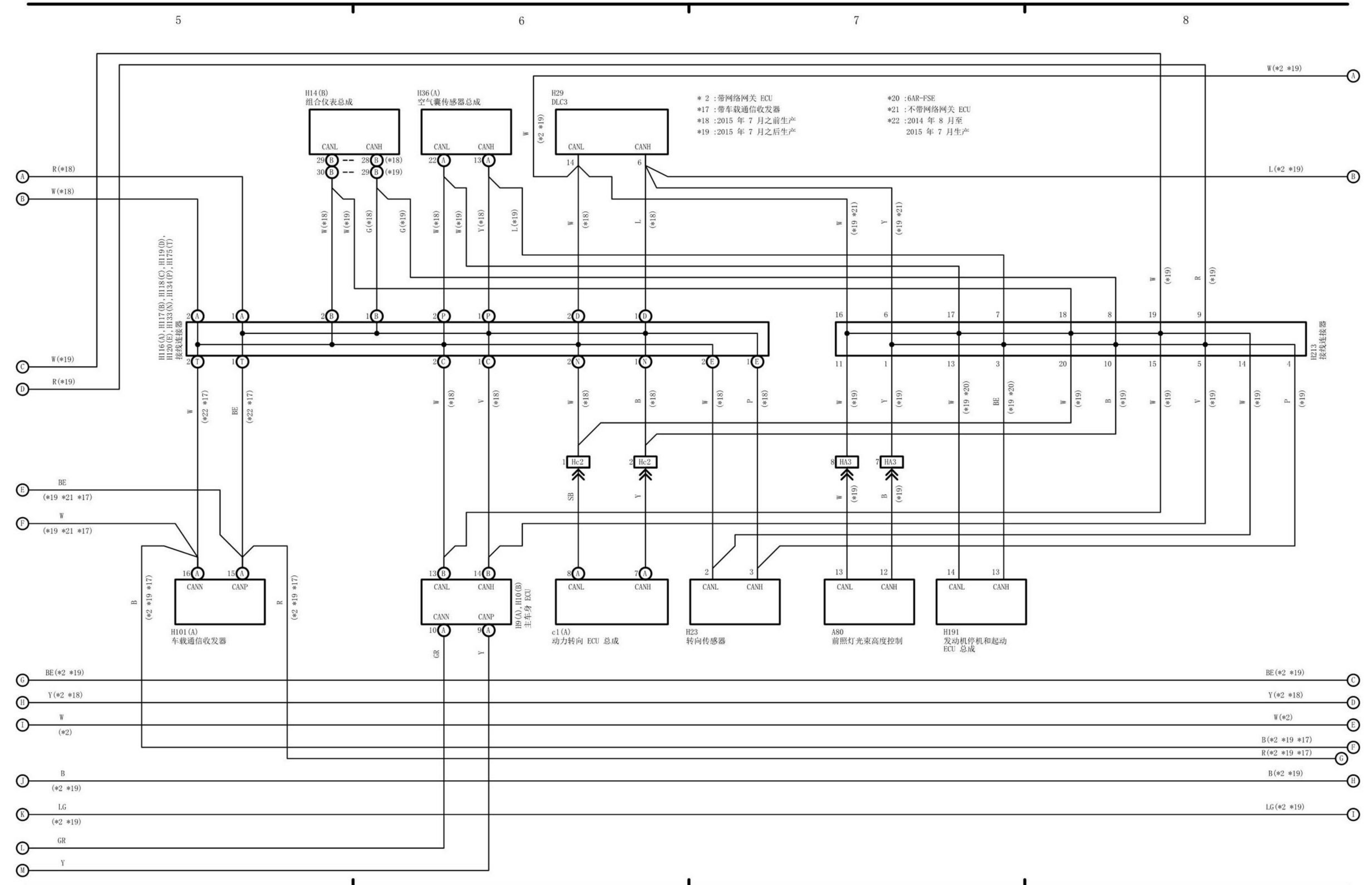
多路通信系统 (CAN) (左驾驶车型)
