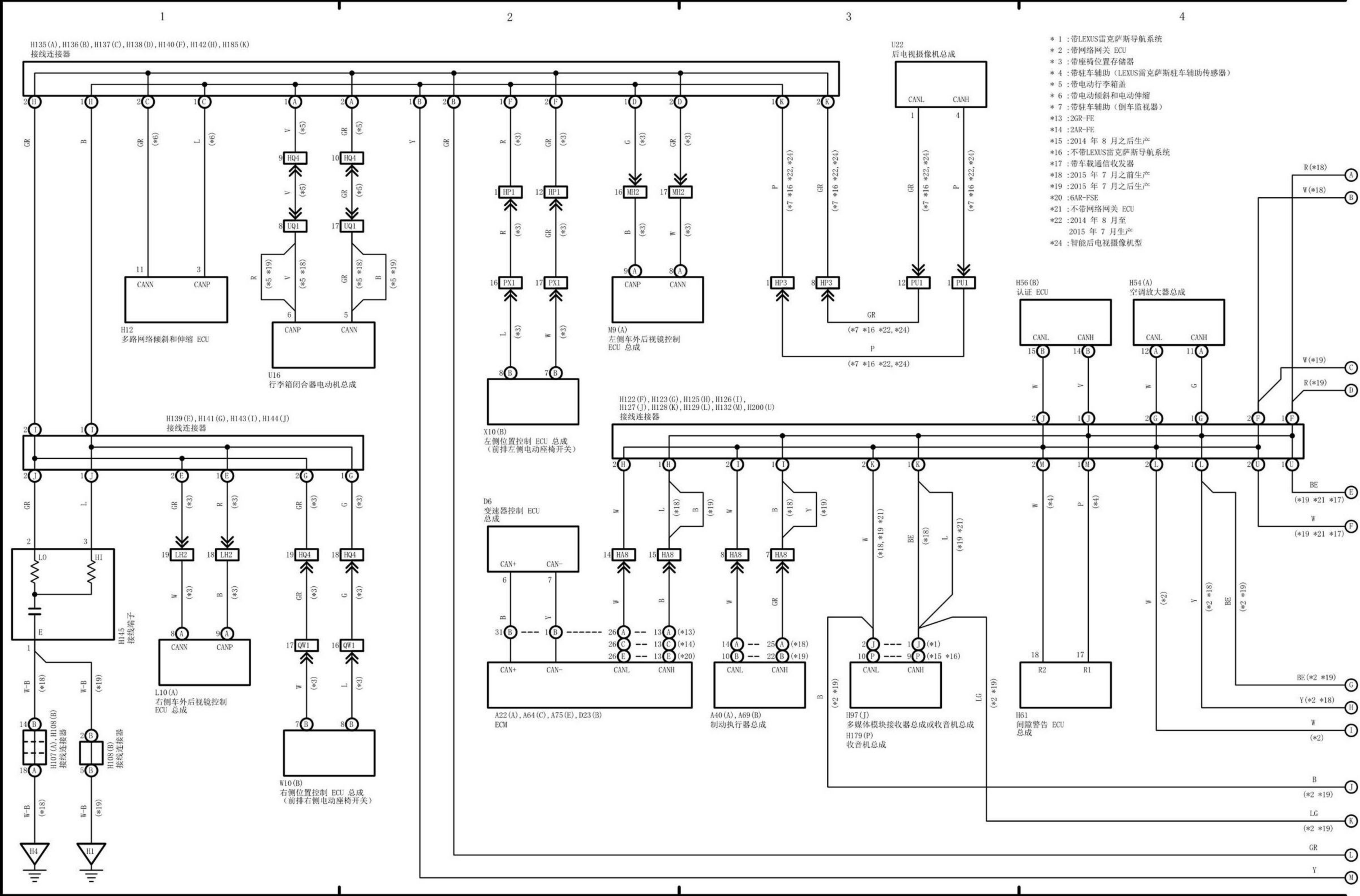
多路通信系统 (CAN) (左驾车型)
